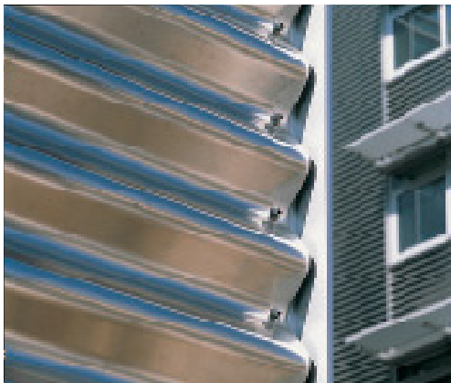
Tôles ondulées en acier inoxydable, fixées à intervalles réguliers par des goujons apparents également en acier inoxydable.
