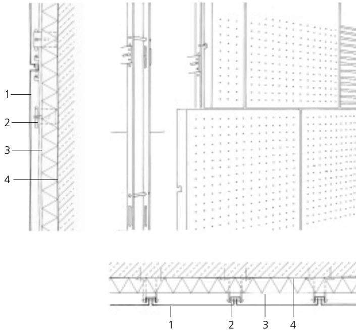
Coupes de la façade
