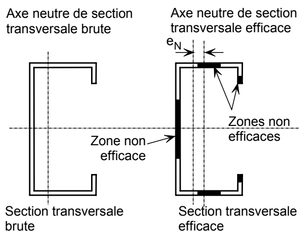
Figure 4.2 Section transversale de Classe 4 comprimée
