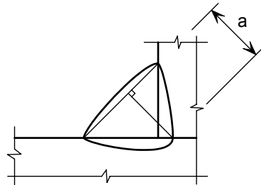
Figure 6.4 Gorge d'une soudure d'angle à forte pénétration
