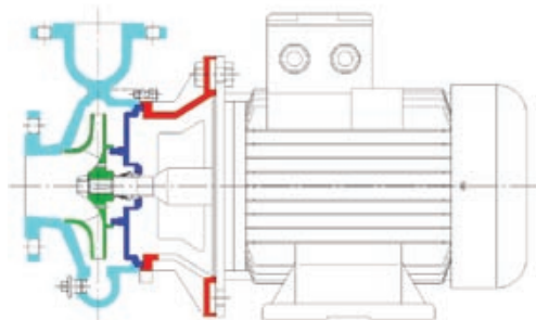
Principaux éléments d'une pompe centrifuge traditionnelle
