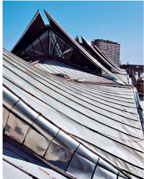
Für das Dach des Gerichtshofes in Antwerpen wurde eine werksseitige 2B-Oberfläche gewählt. Als Werkstoff kam wegen der Meeresnähe die molybdänlegierte Sorte 1.4401 zum Einsatz.
