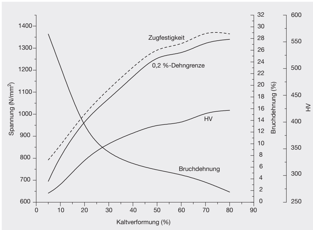
Abbildung 13: Auswirkung der Kaltverfestigung auf die mechanischen Eigenschaften des nichtrostenden Duplexstahls EN 1.4462 (2205) (Quelle: Baosteel)
