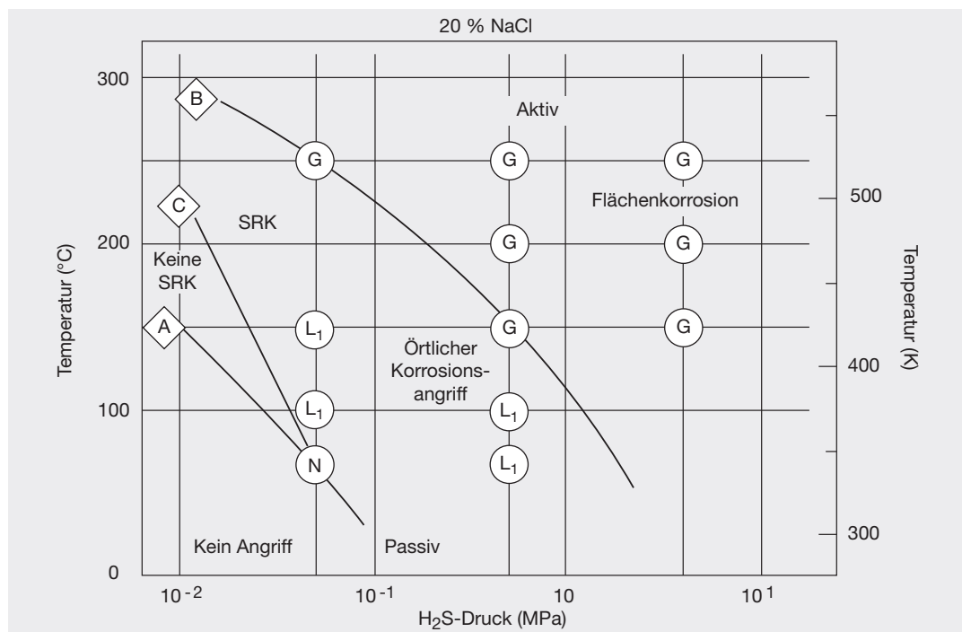
Abbildung 10: Korrosion des nichtrostenden Duplexstahls EN 1.4462 (2205) in 20%iger Natriumchlorid-Schwefelwasserstoff-Umgebung, basierend auf elektrochemischer Vorhersage und experimentellen Ergebnissen
