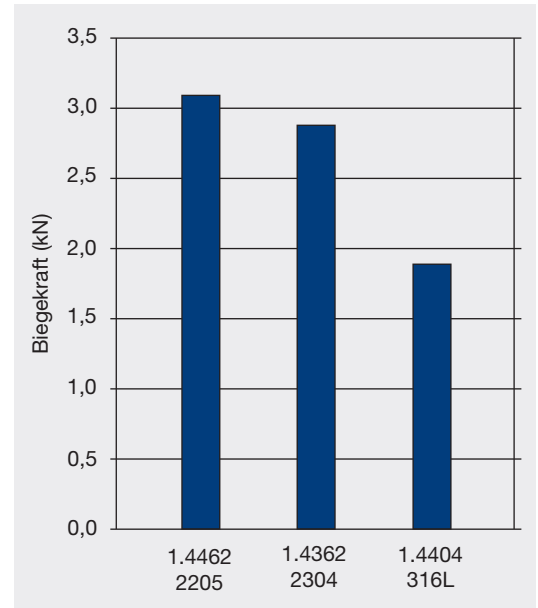
Abbildung 14: Mindestkraft zur Einleitung plastischer Umformung beim Biegen von Proben der Stähle EN 1.4362 (2304), 1.4462 (2205) und 1.4404 (AISI 316 L) mit einer Breite von 50 mm (2 Zoll) und einer Dicke von 2 mm (0,08 Zoll) (Quelle: Outokumpu)
