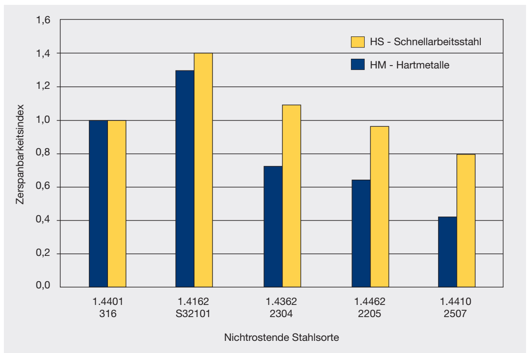
Abbildung 15: Relative Zerspanbarkeit nichtrostender Duplexstähle im Vergleich mit der Sorte EN 1.4401 (AISI 316) mit gesinterten Hartmetallwerkzeugen und für Werkzeuge aus Schnellarbeitsstahl (Quelle: Outokumpu)
