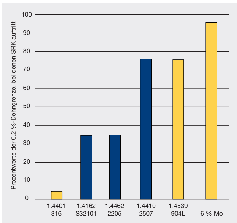
Abbildung 9: Spannungsrisskorrosionsbeständigkeit werksseitig geglähter nichtrostender austenitischer und Duplex-Stähle im Tropfenverdampfungstest mit einer Natriumchloridlösung bei 120 °C (248 °F). Die mechanische Spannung, bei der Spannungsrisskorrosion auftritt, ist in Prozent der 0,2 %-Dehngrenze angegeben (Quelle: Outokumpu)
