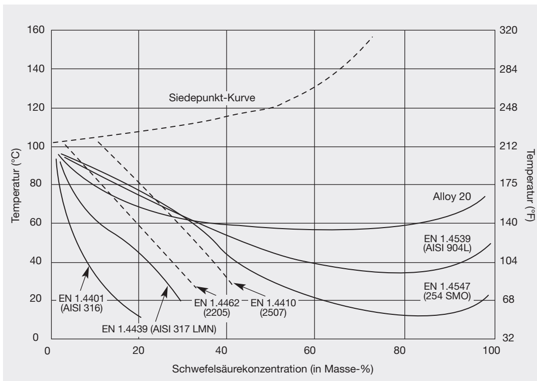
Abbildung 6: Isokorrosionsdiagramm mit 0,1 mm/Jahr (0,004 in/Jahr) Isokorrosionskurven in unbelüfteter Schwefelsäurelösung; Laboruntersuchungen unter Verwendung von p.a. Schwefelsäure (Quelle: Hersteller-Datenblatt, 254 SMO ist ein Markenname von Outokumpu)
