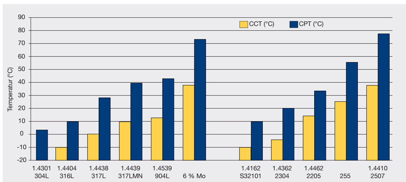
Abbildung 8: Kritische Loch- und Spaltkorrosionstemperaturen (KLT und KST) für ungeschweißte austenitische (links) und Duplexstähle (rechts) im lösungsgeglühten Zustand (gemessen in 6%iger Eisenchloridlösung gemäß ASTM G 48)
