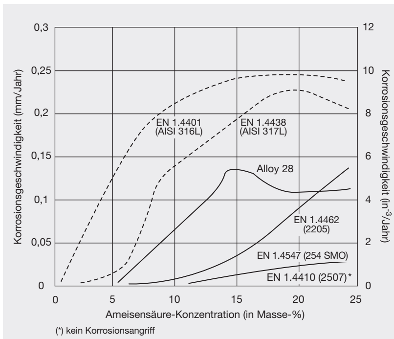
Abbildung 7: Korrosion bei austenitischen und Duplex-Stählen in siedenden Lösungen von 50 %iger Essigsäure mit zunehmenden Anteilen an Ameisensäure (Quelle: Sandvik)
