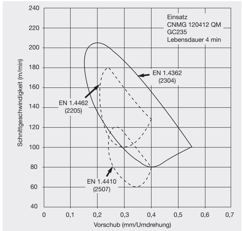
Abbildung 16: Vergleich der Zerspanungsparameter für das Drehen von nichtrostenden Duplexstählen mit gesintertem Hartmetalleinsatz bei einer Werkzeug-Lebensdauer von vier Minuten (Quelle: Sandvik)
