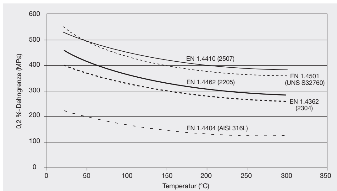
Abbildung 11: Vergleich typischer 0,2 %-Dehngrenzen von nichtrostenden Duplexstählen und dem Stahl EN 1.4404 (AISI 316L) zwischen Raumtemperatur und 300 °C (Quelle: Produktdatenblatt)
