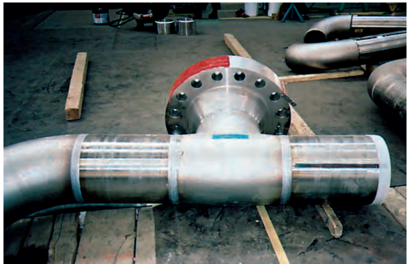
Geflanschte T-Verbindung aus dem Werkstoff EN 1.4462 (2205); (Quelle: Arco Exploration and Production Technology)
