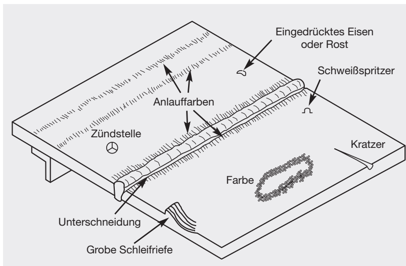
Abbildung 18: Häufig anzutreffende Verarbeitungs- oder Oberflächenfehler (Quelle: Nickel Institute Publication 10 026)
