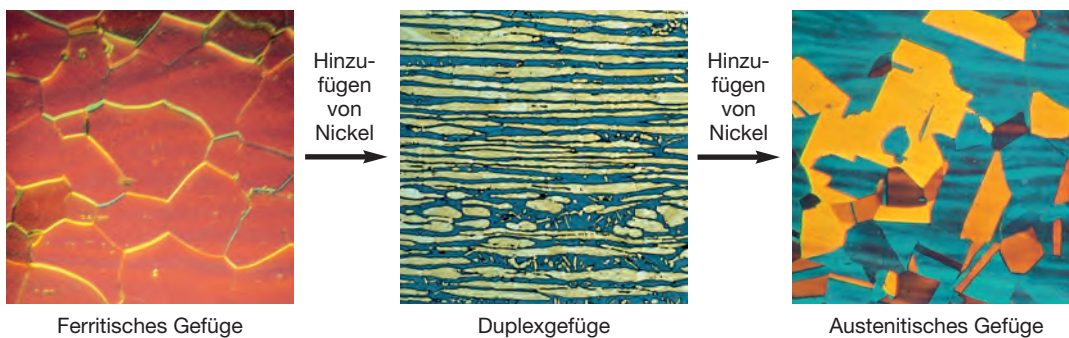
Abbildung 2: Durch Erhöhung des Nickelgehaltes verändert sich das Gefüge der nichtrostenden Stähle von ferritisch (links) über austenitisch-ferritisch (Mitte) zu austenitisch (rechts). Die Aufnahmen zeigen polierte und geätzte Proben unter einem Lichtmikroskop. Innerhalb des Duplex-Gefüges wurde der Ferrit eingefärbt, so dass er als die dunklere Phase erscheint. (Quelle: Outokumpu)
