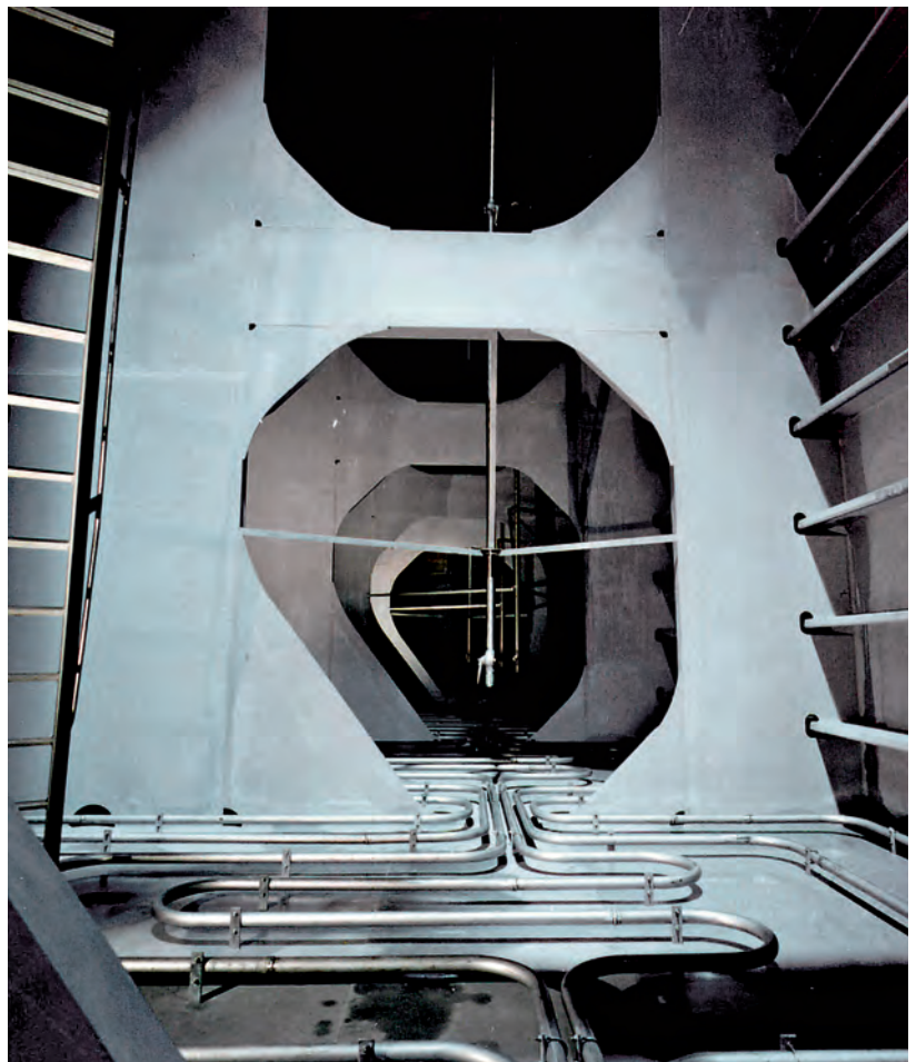
Chemikalienanker; Innenansicht des Tanks aus dem Werkstoff EN 1.4462 (2205); (Quelle: ThyssenKrupp Nirosta)
