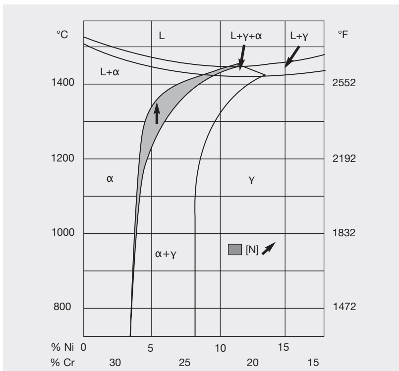
Abbildung 3: Schnitt durch das ternäre Fe-Cr-Ni-Phasendiagramm bei 68 % Eisen: bereits geringe Änderungen im Chrom- und Nickelgehalt wirken sich stark auf das Gleichgewicht von Austenit und Ferrit in nichtrostenden Duplexstählen aus.
