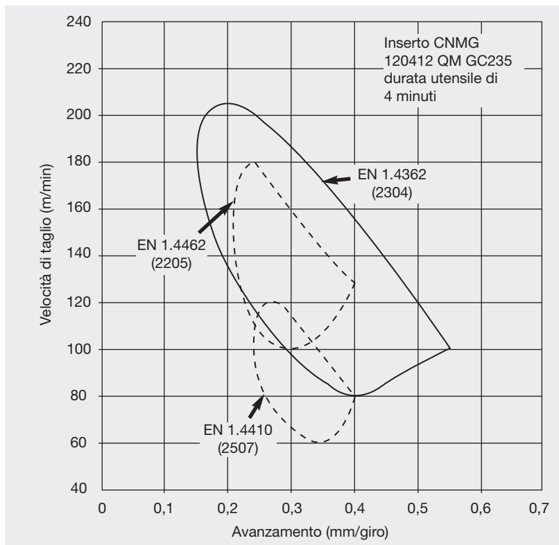
Figura 16: Confronto tra i parametri di lavorazione per la tornitura di acciai duplex con inserti in carburo cementato con una durata dell'utensile di quattro minuti (Fonte: Sandvik)
