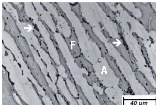
Figura 4: Microstruttura di un campione di EN 1.4462 (2205) trattato ad 850 °C (1560 °F) per 40 minuti con precipitazione di fase sigma (frecce) in corrispondenza dei bordi grano tra ferrite ed austenite. La fase ferritica (F) appare più scura rispetto a quella austenitica (A) nella micrografia (Rif. 3).
