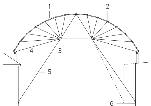
Sezione trasversale scala 1:250
