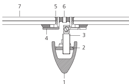
Sezione orizzontale scala 1:5
