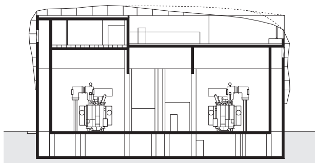
Sezione trasversale, scala 1:500
