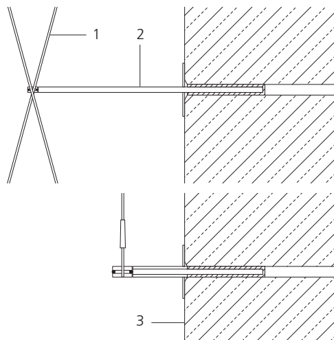
Sezione verticale, scala 1:10
